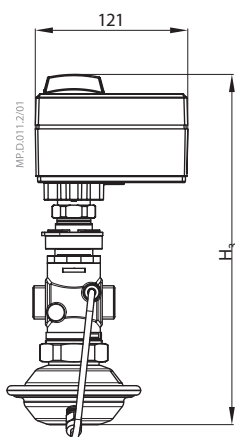
AMV(E) 10 + AVQM (DN 15)
