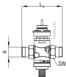
AMV(E) 13 + AVQM (DN 15)
