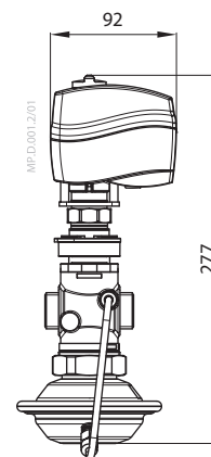
AMV 150 + AVQM (DN 15)
