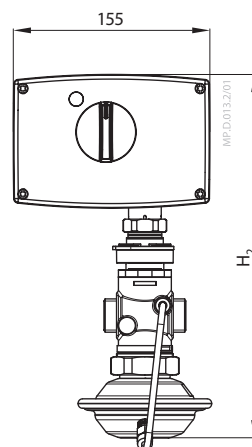
AMV(E) 2./3. + AVQM (DN 15-32)
